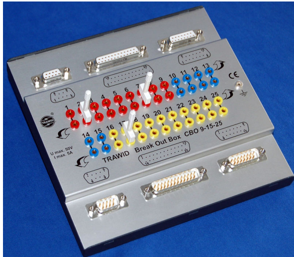
Break Out Box für D-Sub Steckverbindungen 9-polig, 15-polig, 25-polig. Ausführung s. Standard. Abmessungen: 176 x 172 x 30 (mm) Gewicht: 615 g
