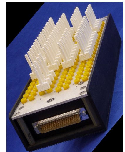
Break Out Box im Al-Gehäuse bis 78-polig. D-Sub Stecker und D-Sub HD Stecker handverdrahtet. Andere Steckverbinder auf Anfrage.
