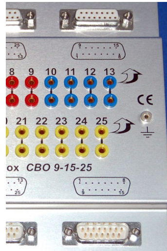
Break Out Box für D-Sub Steckverbindungen 9-polig, 15-polig, 25-polig. Ausführung s. Standard. Abmessungen: 176 x 172 x 30 (mm) Gewicht: 615 g
