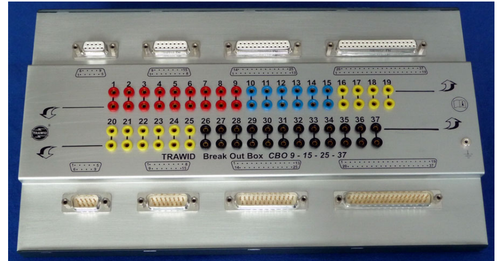
Break Out Box für D-Sub Steckverbindungen 9-polig, 15-polig, 25-polig, 37 polig. Ausführung s. Standard. Abmessungen: 296 x 172 x 30 (mm) Gewicht: 880 g
