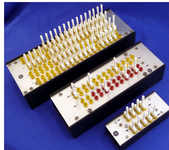
Break Out Box im Al-Gehäuse bis 78-polig. D-Sub Stecker und D-Sub HD Stecker handverdrahtet. Andere Steckverbinder auf Anfrage.
