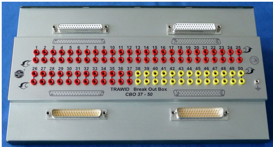
Break Out Box für D-Sub Steckverbindungen 37-pol., 50-pol. Ausführung s. Standard. Abmessungen: 296 x 172 x 30 (mm) Gewicht: 1040 g
